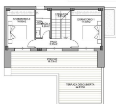
PLANTA PRIMERA
