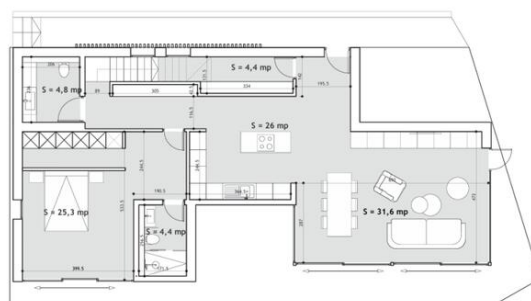
PLANTA BAJA
