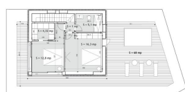
PLANTA ALTA
